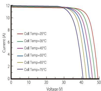
温度特性 (I-V) : LR4-72HPH-440M
