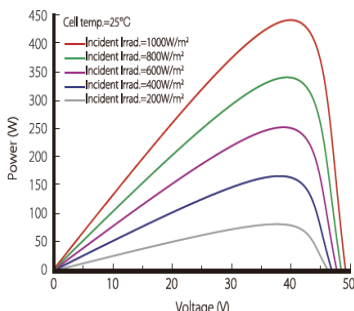
放射照度特性 (P-V) : LR4-72HPH-440M
