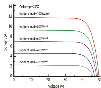
放射照度特性 (I-V) : LR4-72HPH-440M
